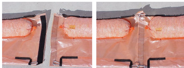
Verbinden der Sektionen mit Schnellkupplung
